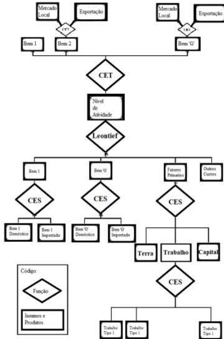
Figura 1 – Fluxograma do modelo ORANI
