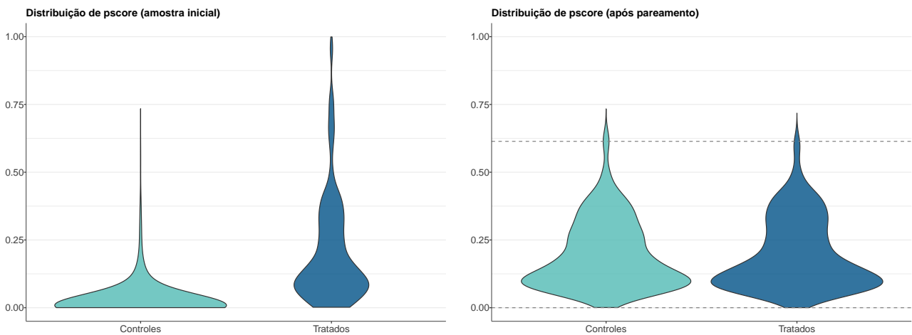
Figura 3: Distribuição do p -score entre grupos de tratamento e de controle e limites da região de suporte comum (amostra original e após pareamento)
