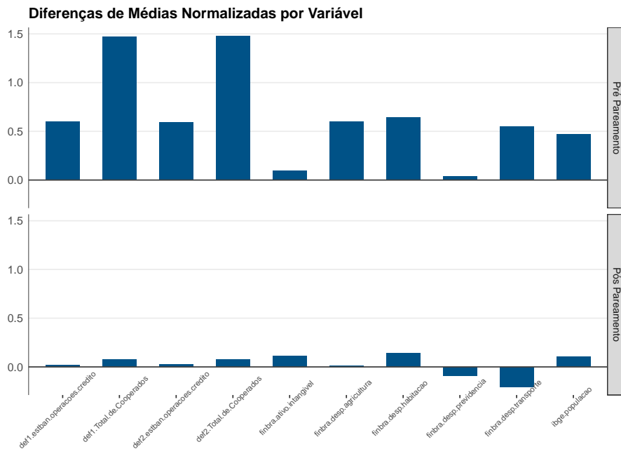
Figura 2: Diferenças de Médias Normalizadas das Variáveis de Controle
