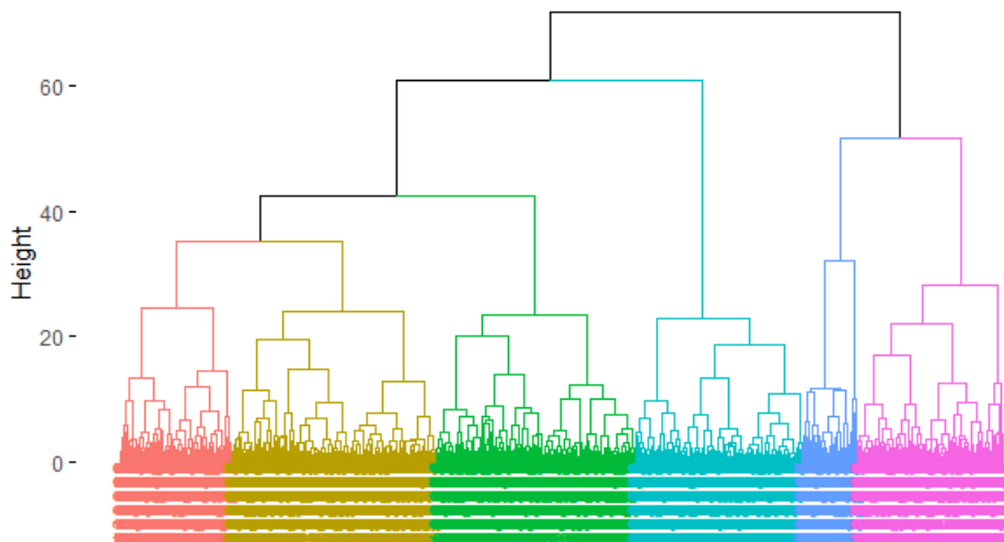
Figura 3 – Dendograma
