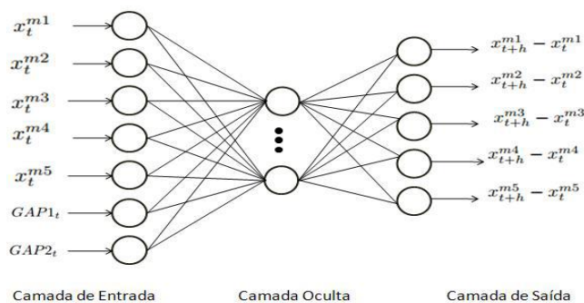
Figura 1: Arquitetura Rede Neural Estática.
